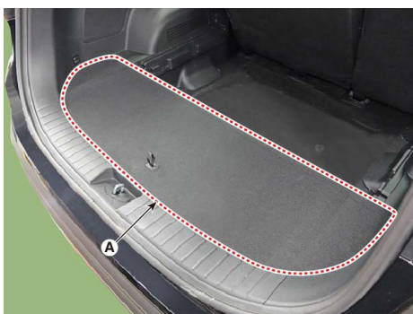
4-1. Remove the luggage mat(A).
